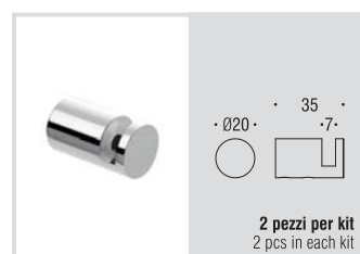
TKIT/04 Ferma pannelli frontale per spessore max 7mm Front-type kit for thickness max 7mm
